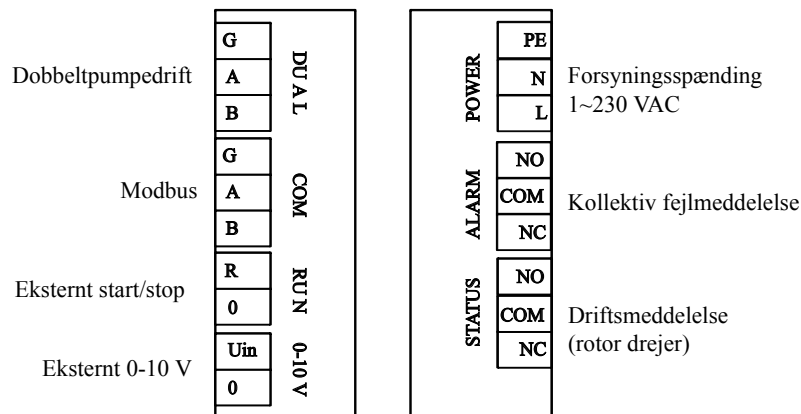
III. 10: Tilslutningsdiagram Magneta D Smedegaard 40-120/-180, 50-100/-120 og 65-80/-120
