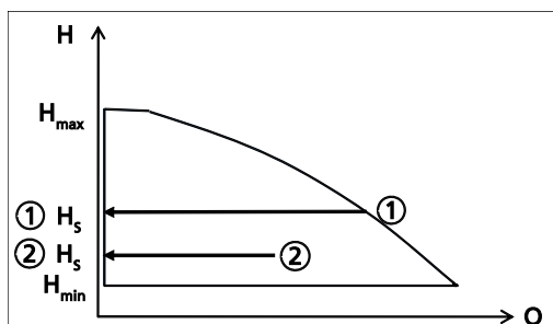
III. 16: Konstantrykreguleringens funktion
