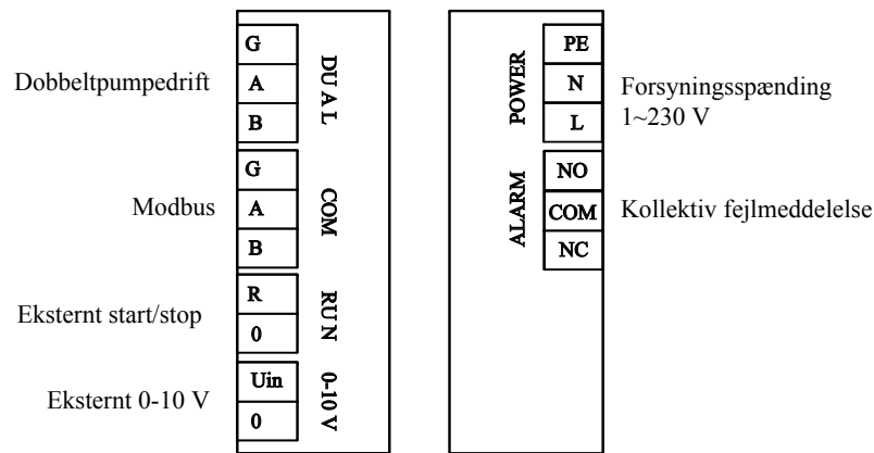
III. 9: Tilslutningsdiagram Magneta D Smedegaard 30-60/-100, 32-80/-120, 40-80/-100 og 50-80 7)
