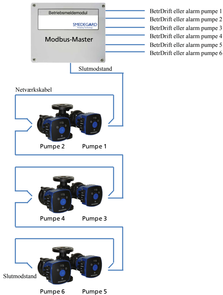
III. 11: Tilslutning af pumper Magneta D Smedegaard til driftsmeddelelsesmodul 01550860
