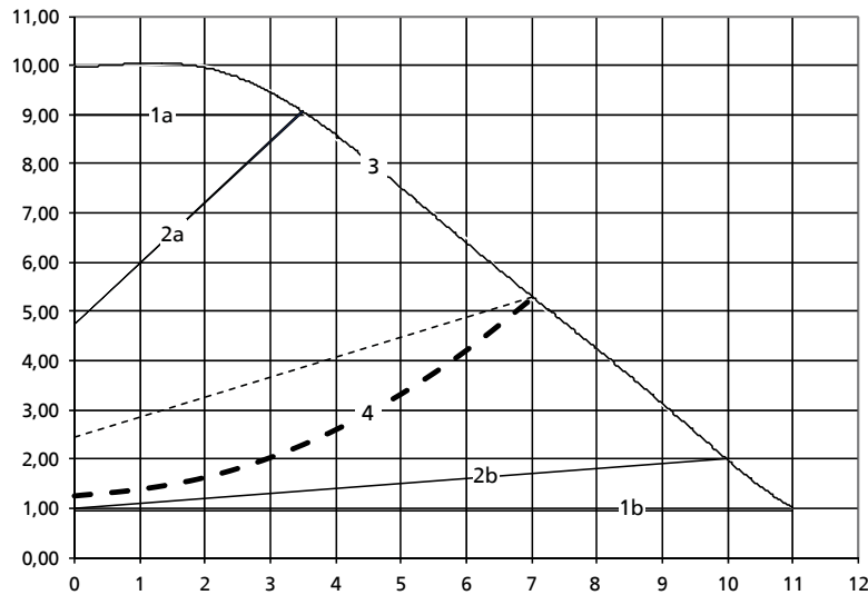
III. 25: Eco-mode – kurve med pumpe i størrelsen 25-100 som eksempel
