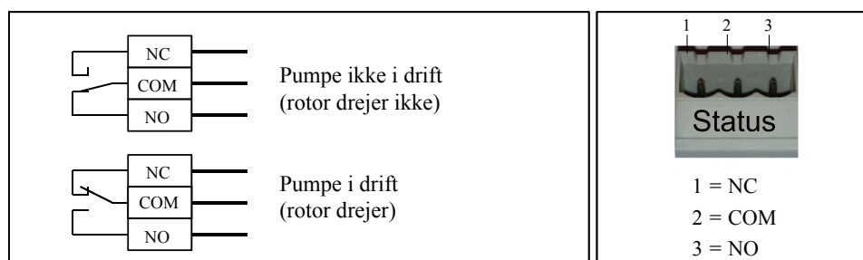
III. 34: Tilslutningsdiagram driftsmeddelelse
