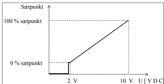
Ill. 27: Analogt signal 0-10 V som nominel værdi for pumpen
