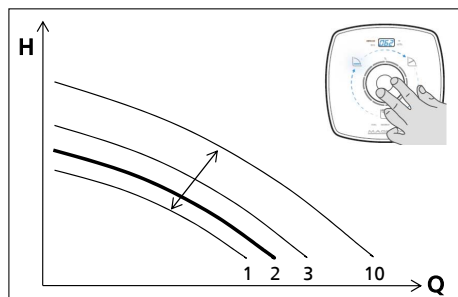
III. 23: Indstilling af drift med fast omdrejningstal
