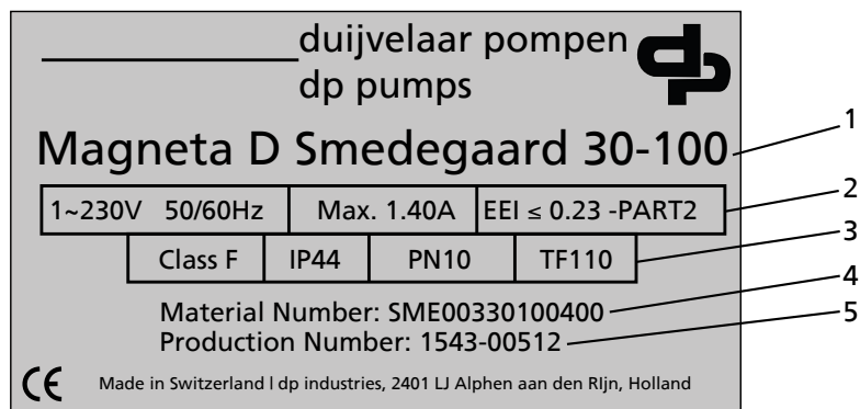
Ill. 4: Typeskilt (eksempel)
