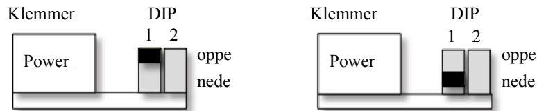
III. 29: Stilling DIP-kontakt 1
