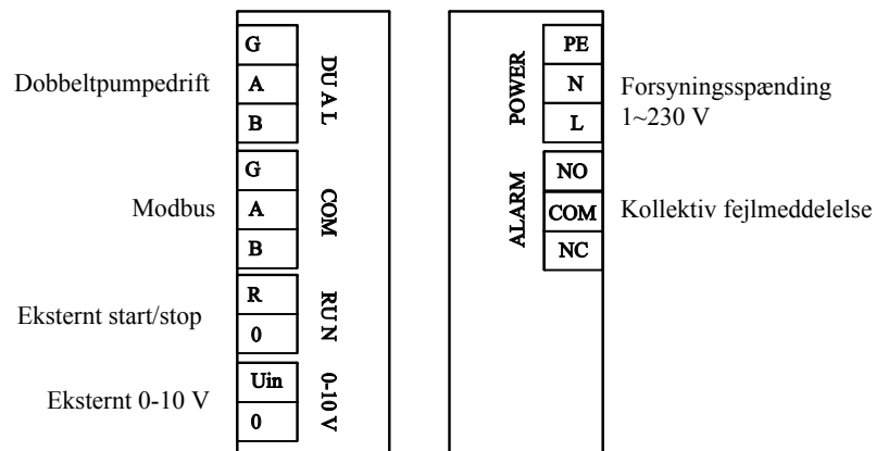
III. 35: Elektrisk tilslutningsplan Magneta D Smedegaard 30-60/-100, 32-80/-120, 40-80/-100 og 50-80 9)
