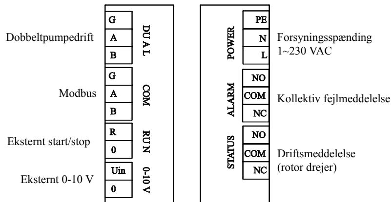
III. 36: Elektrisk tilslutningsplan Magneta D Smedegaard 40-120/-180, 50-100/-120 og 65-80/-120
