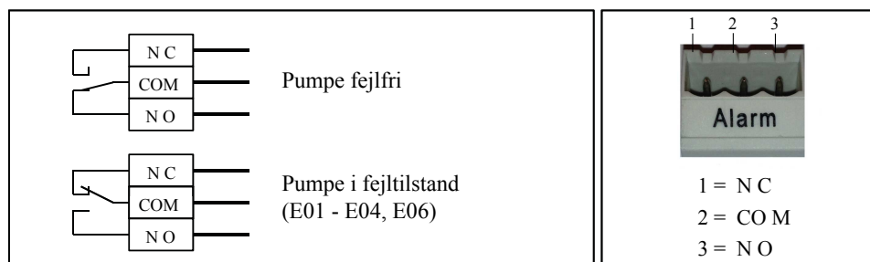
III. 33: Tilslutningsdiagram alarmmeddelelse
